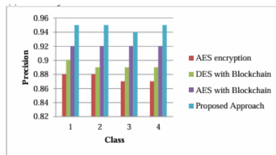
(b) Precision
